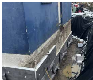
DRENERING OG ETTERISOLERING
